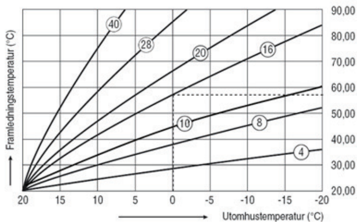
Kurvlutning vid 20°C önskad rumstemperatur.
